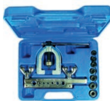
Przyrząd do zarabiania przewodów
